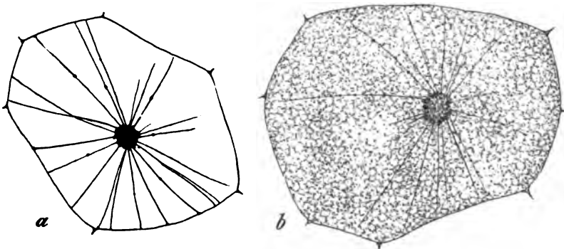
Fig. 12. Strahlungen und gröber maschige Gerüste, entstanden durch Fällung einer Mischung von 5-proc. Albumose und 2,5-proc. Hämoglobin, leicht sauer, durch 1-proc. Osmiumsäure in Hollundermarkschnitten. Diese waren nicht gleich reichlich in allen Zellen injicirt und daher entstanden theils reine Strahlungen um den Kernrest ( a ), theils wurden sie eingebettet in das maschige Gerüst, das sie theilweise verdeckt, theilweise aber ungetrübt bis an die Zellwand hervortreten lässt ( b ). Aus welchem Stoff hier die Strahlungen und Gerüste bestehen, ob aus den beiden Gemischcomponenten oder nur aus einer, ist nicht sicher zu sagen. Die Strahlungen sind hier sehr schön homogen-fädig, stellenweise knotig angeschwollen durch kleine Vacuolen, die infolge partieller Wiederlösung der Strahlensubstanz in dem Fixierungsmittel sich gebildet hatten. (Vergr. a und b 600.)
